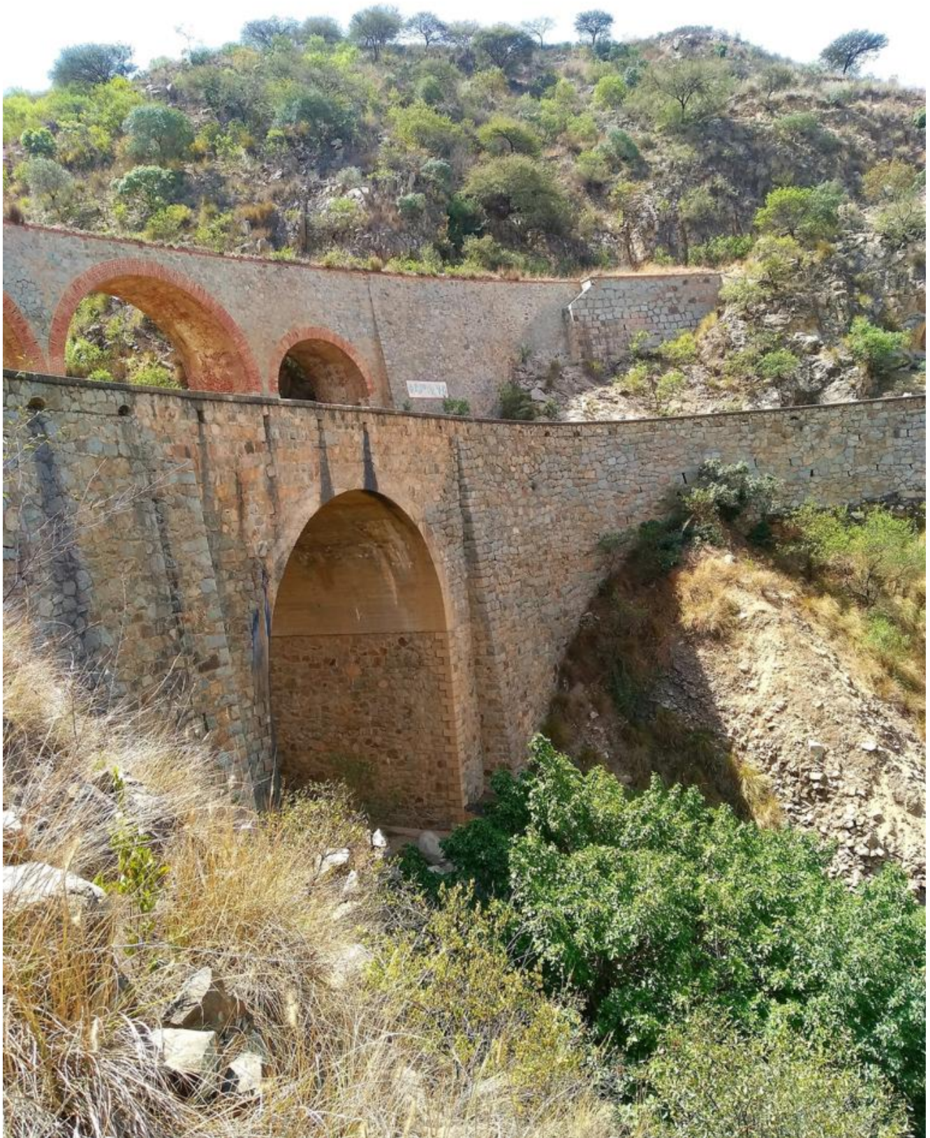
Viadukt Eritrea
